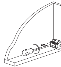
Skapja regulējams balsts stiprinās pie cokola ar kronšteinu
